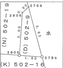
拡大図 K 縮尺150分の1
