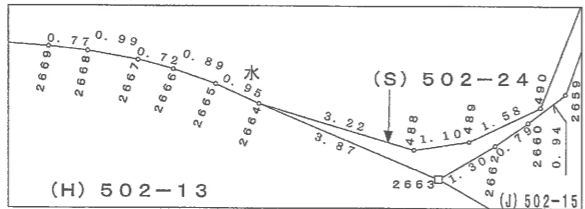
拡大図 二 縮尺150分の1
