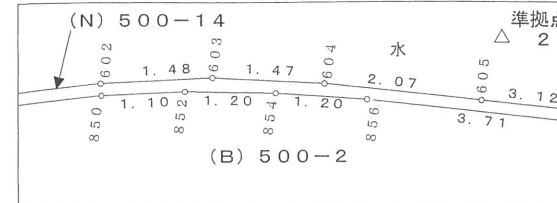
詳細図 ヘ 1:100
