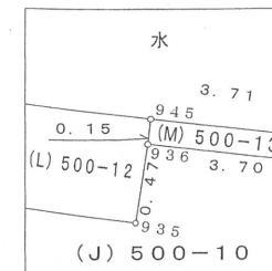
詳細図 イ 1:50
