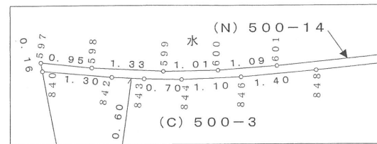
詳細図 ホ 1:100
