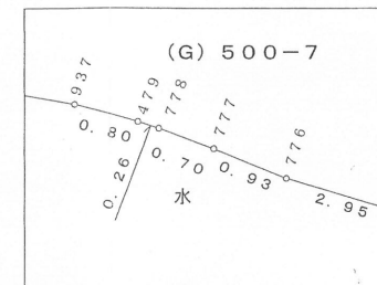
詳細図 ケ 1:100
