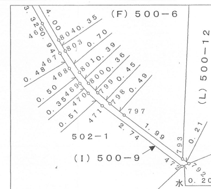
詳細図 コ 1:100
