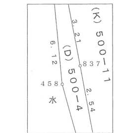
詳細図 ニ 1:100
